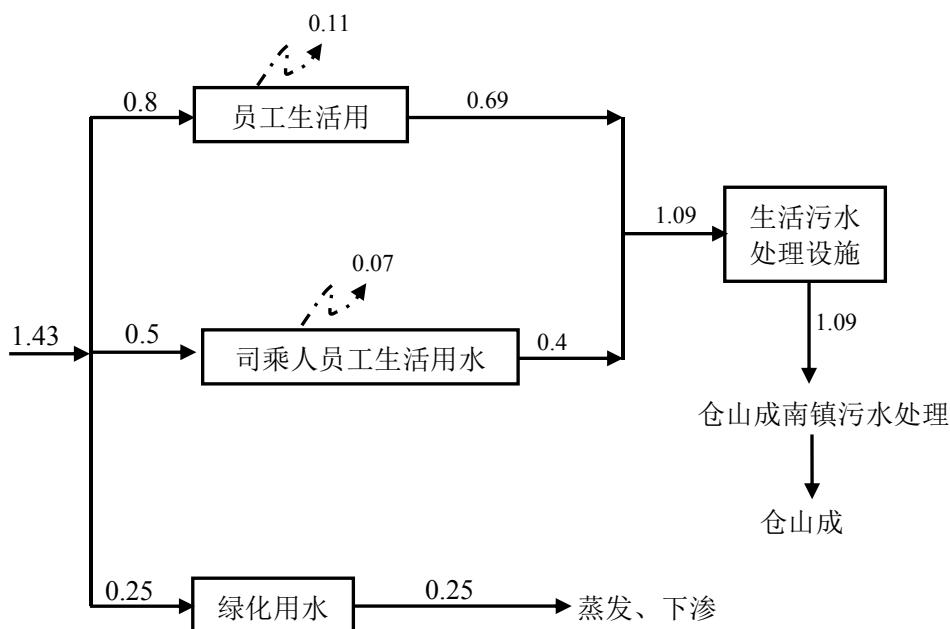
图 2-1 本项目水平衡图 单位：t/d
